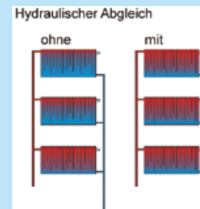
HK: Schema hydraulischer Abgleich
